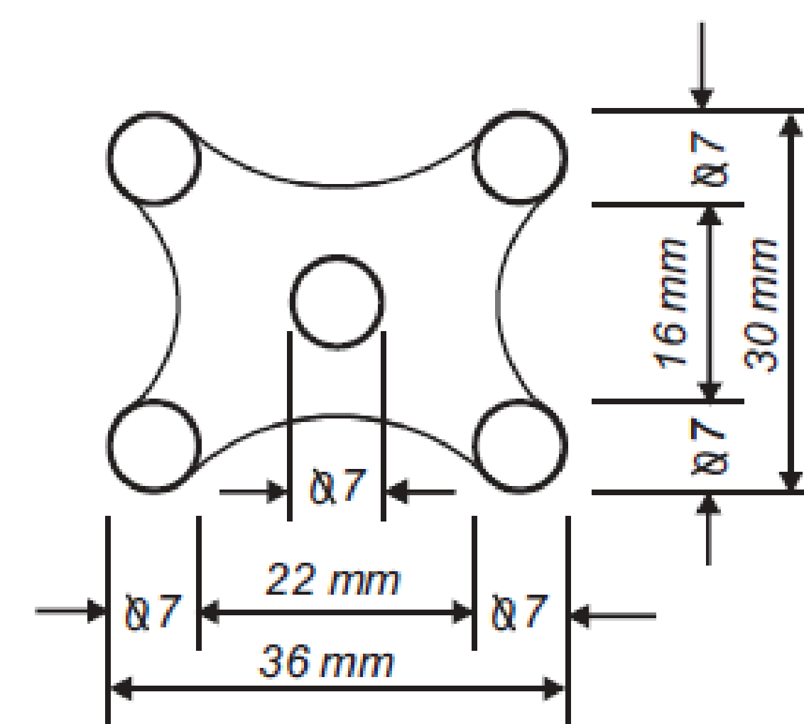
VISTA SUPERIOR
