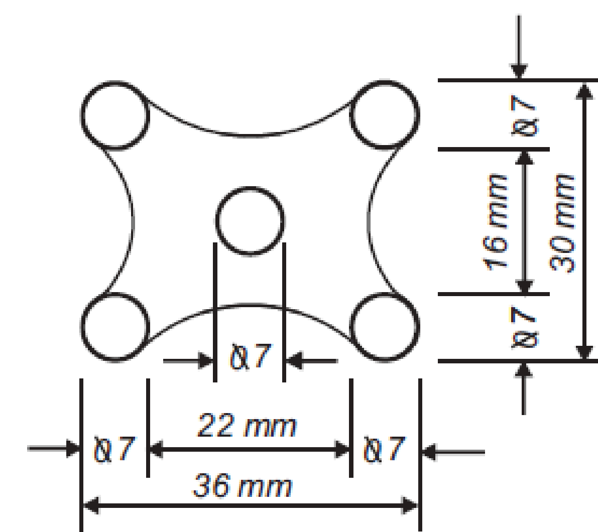
VISTA SUPERIOR
