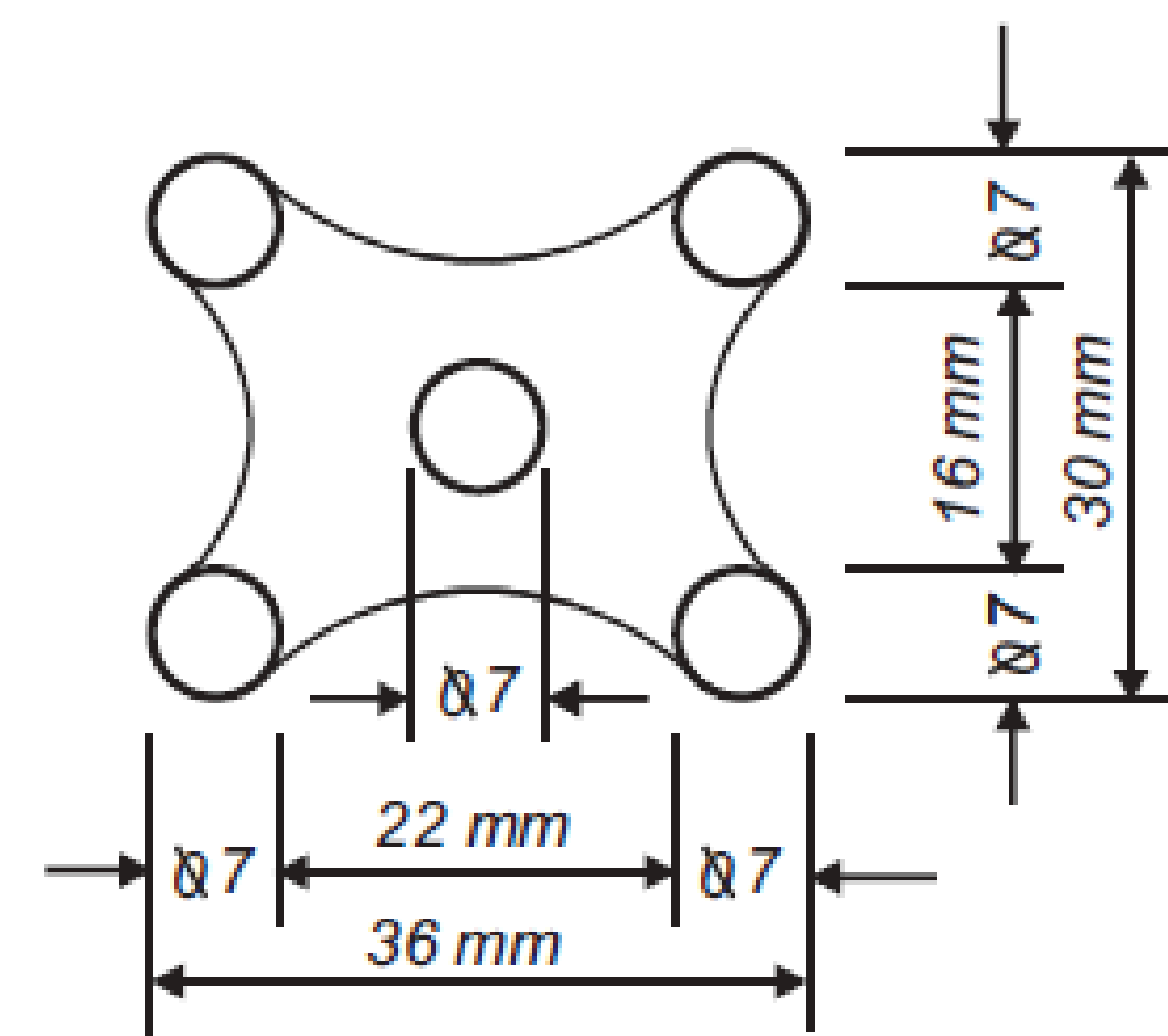
VISTA SUPERIOR
