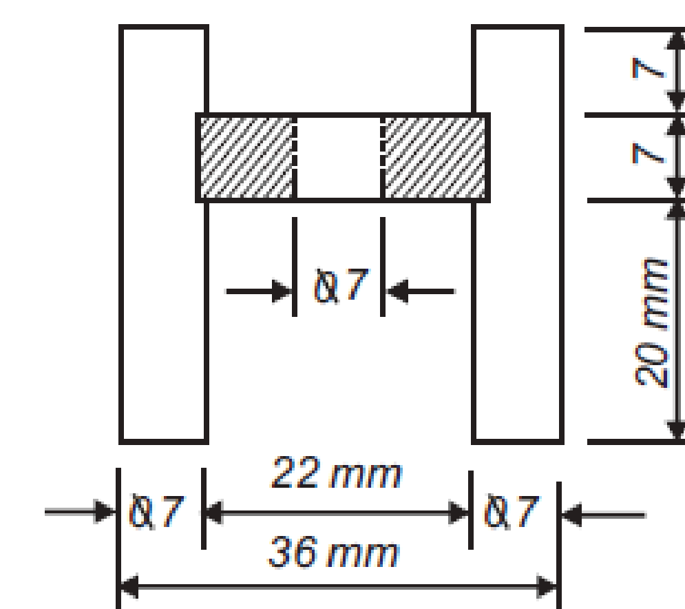
CORTE A-B
