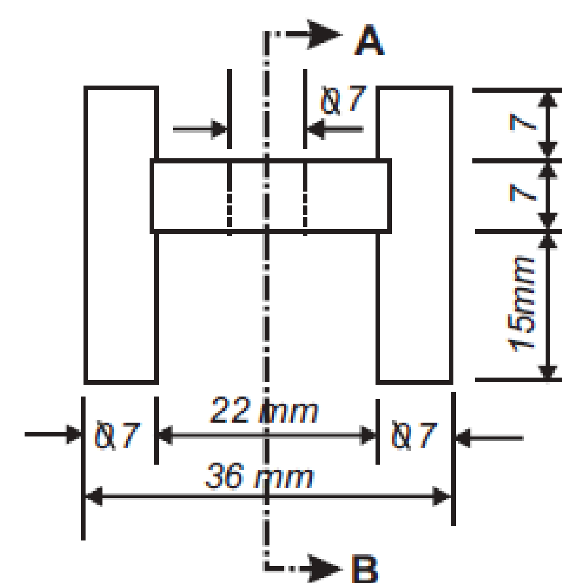
VISTA LATERAL
