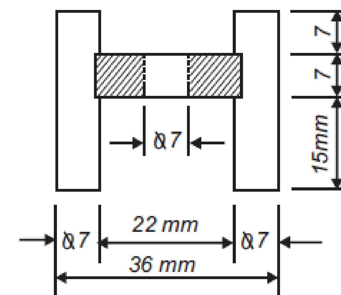
CORTE A-B
