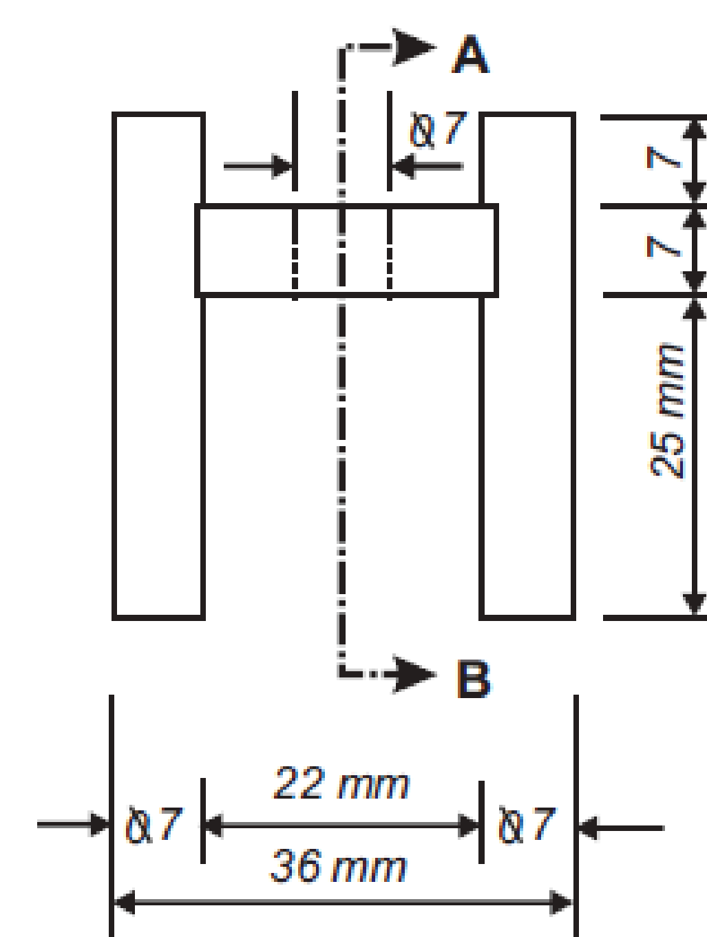
VISTA LATERAL
