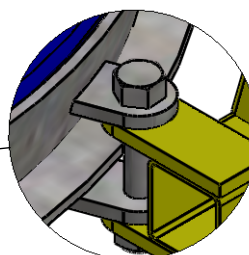
DETALHE H ESCALA 1 : 3
